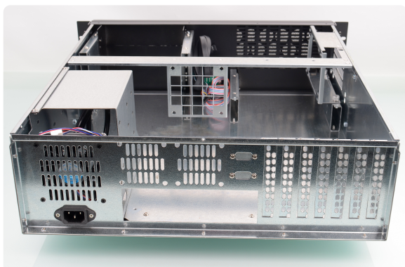
Промышленный корпус IPCWAY Уран-480 (430x133x480)
